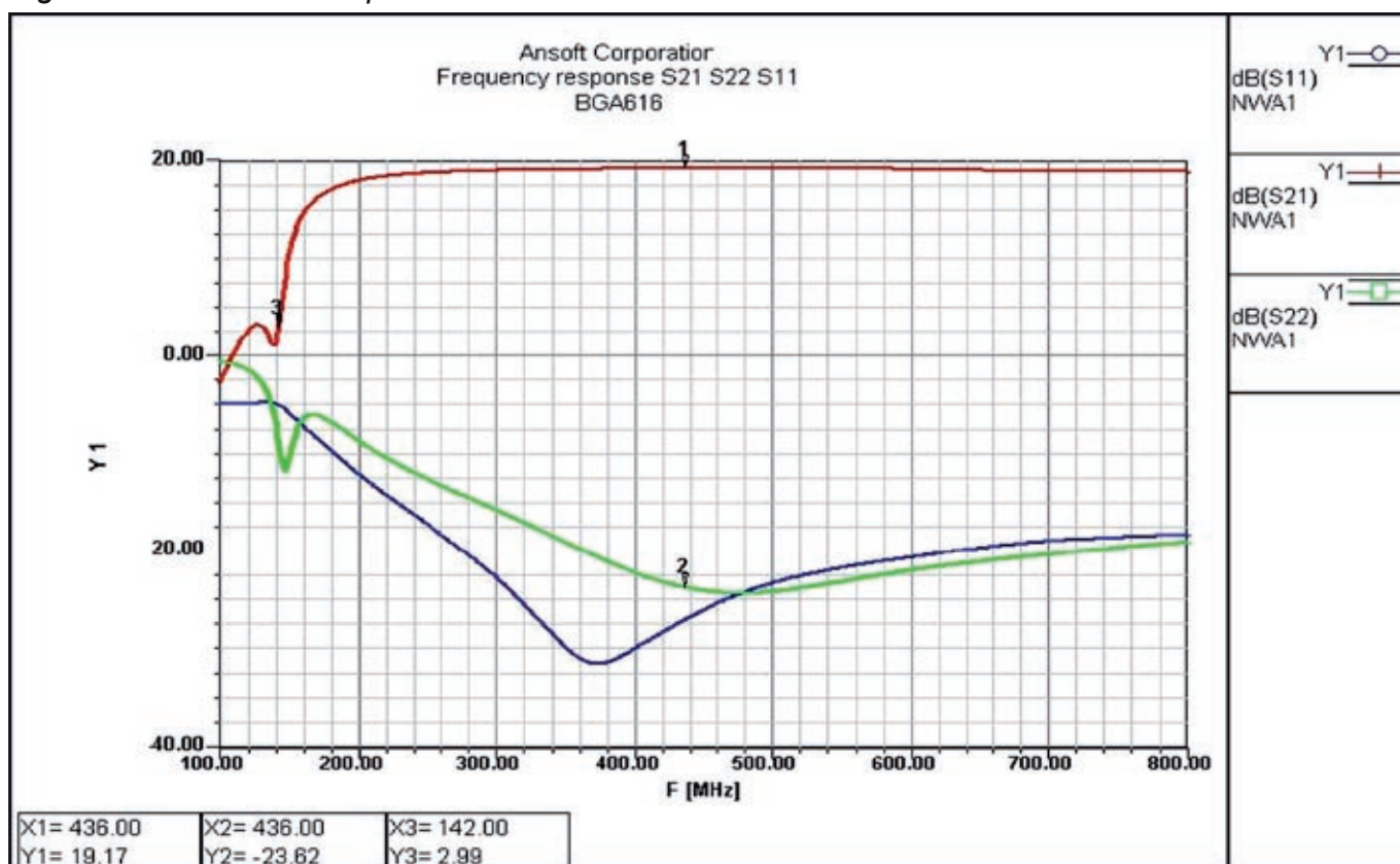
Figure 9 : Simulation amplificateur avec le BGA616 : +19 dB
