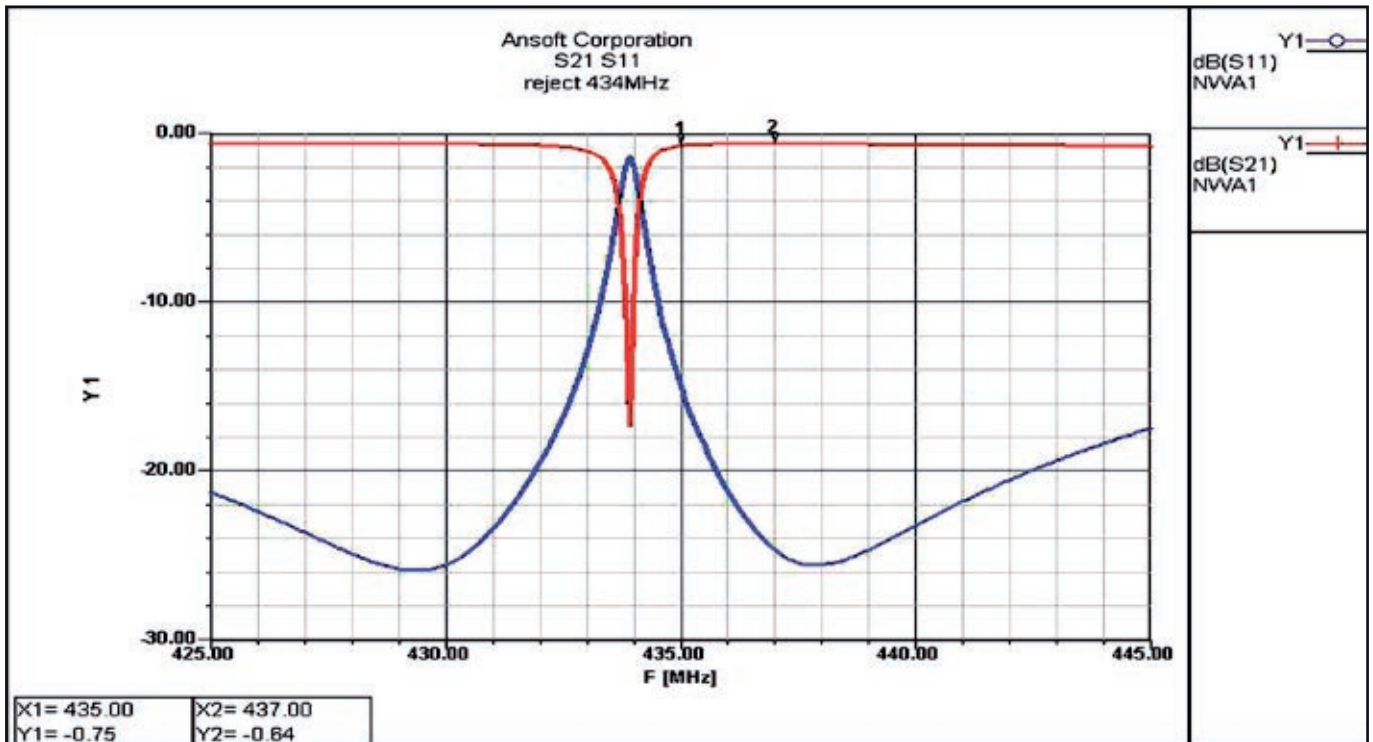
Figure 7 : Simulation du filtre réjecteur centré sur 433.92 MHz.
