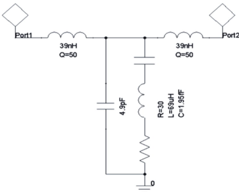
Figure 6 : Schéma de principe du réjecteur pour étude en simulation.
