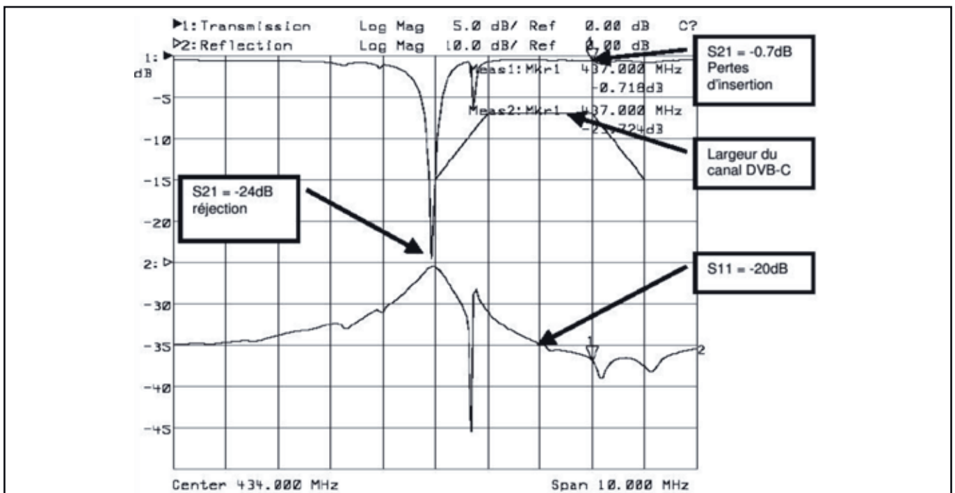
Figure 8 : Application pratique d'un résonateur à ondes de surface en filtre réjecteur à 433.92MHz.
